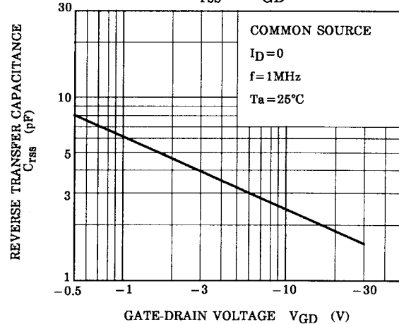
C_{rss} - V_{GD}
