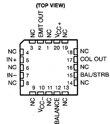
LM111 . . . FK PACKAGE
