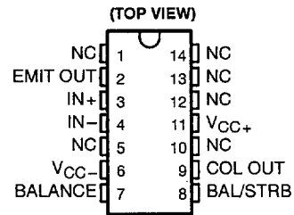
LM111 . . . JG PACKAGE LM211, LM311 . . . D, DB, P, OR PW PACKAGE
