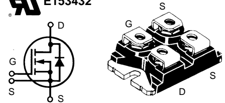
miniBLOC, SOT-227 B E153432
