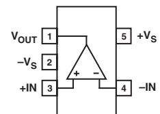
SC70 (KS) AD8033
